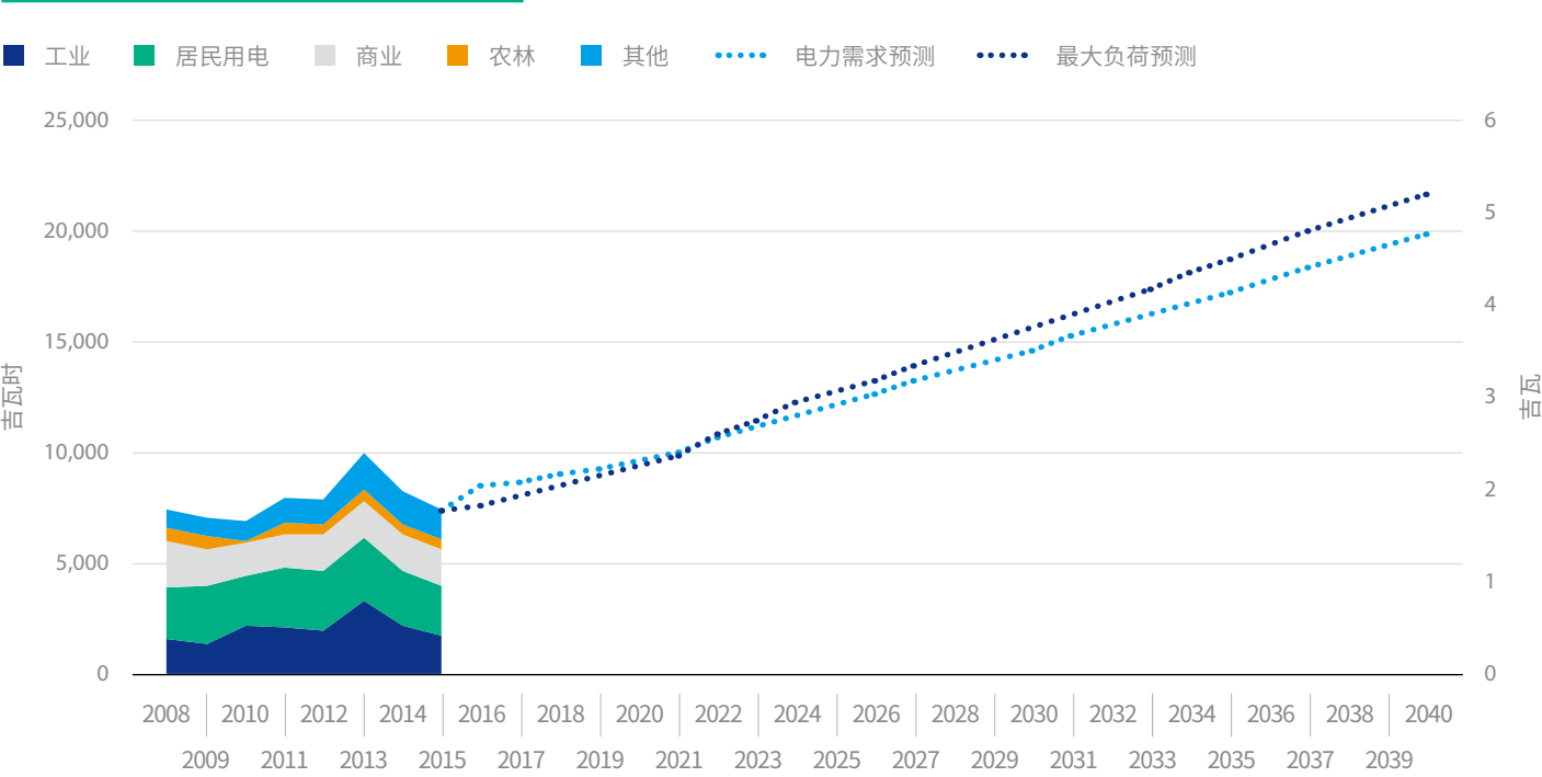
图 20. 津巴布韦电力需求及最大电力负荷
