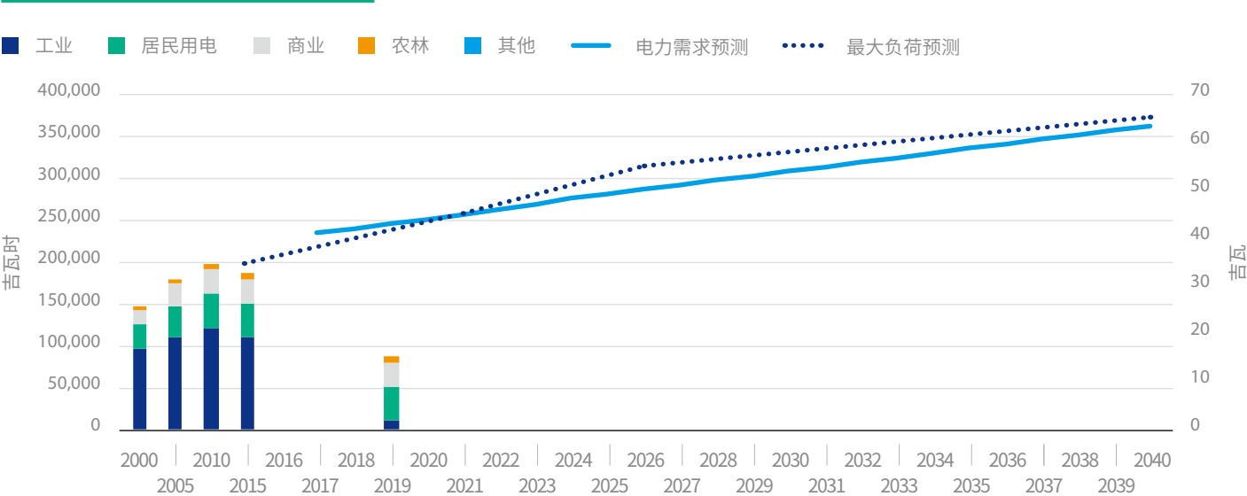
图 25. 南非电力需求及最大电力负荷
