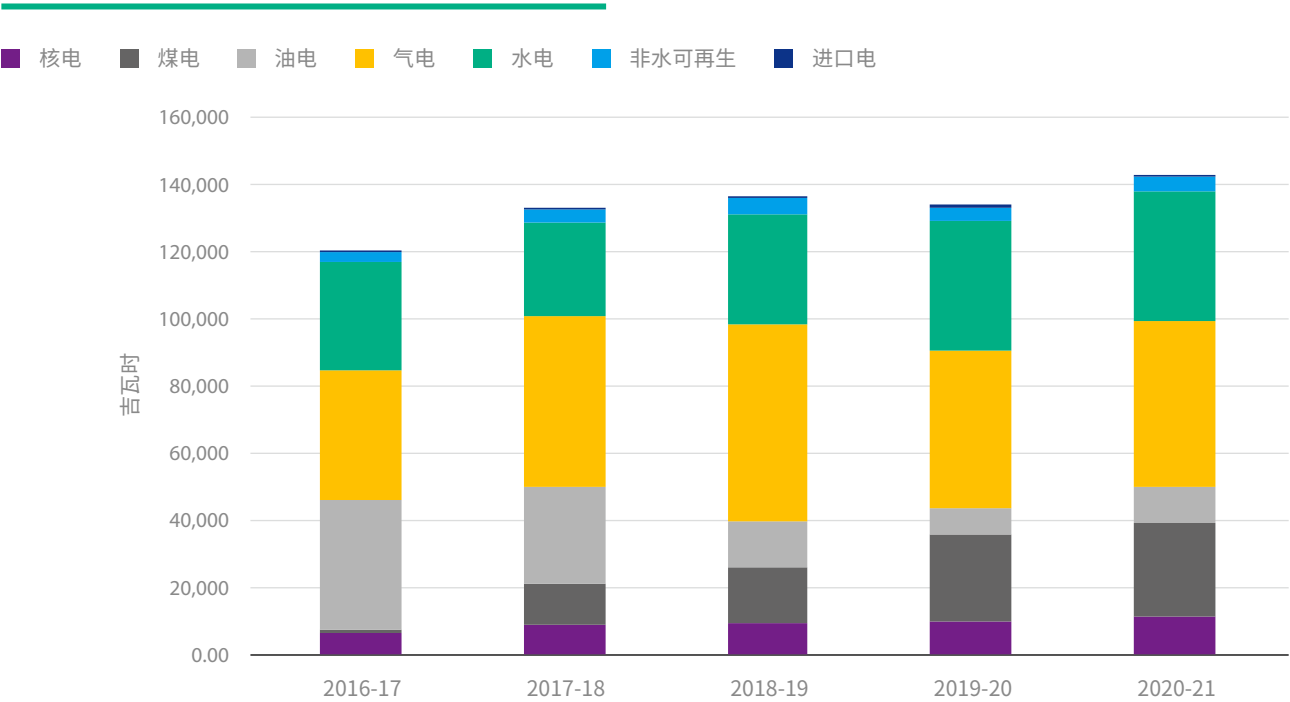
图 14. 巴基斯坦发电量及结构变化（2016年-2021年）
