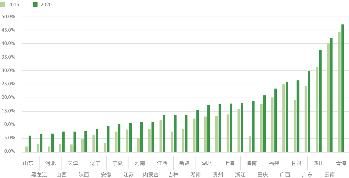
图 12. 非化石能源占比（%）
