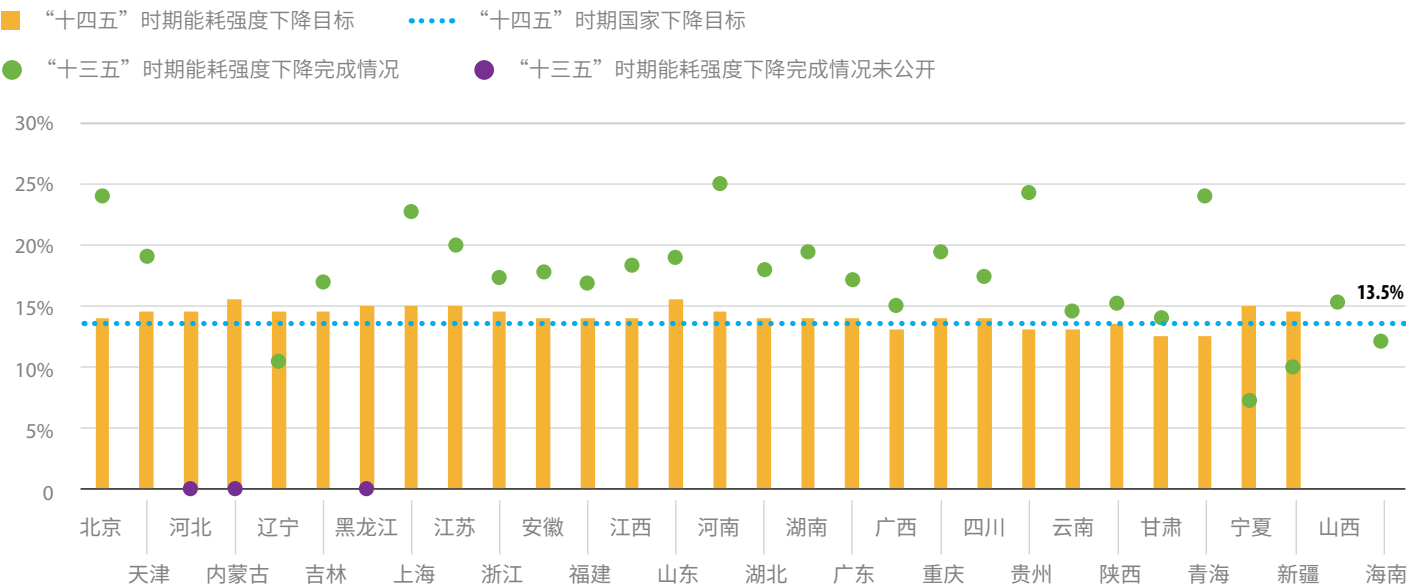
图 19. 各省级地区“十四五”时期能耗强度下降目标
