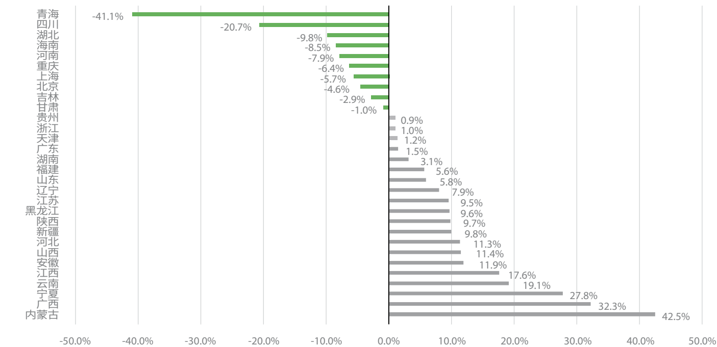
图 8. 2015-2020年人均能源相关碳排放变化
