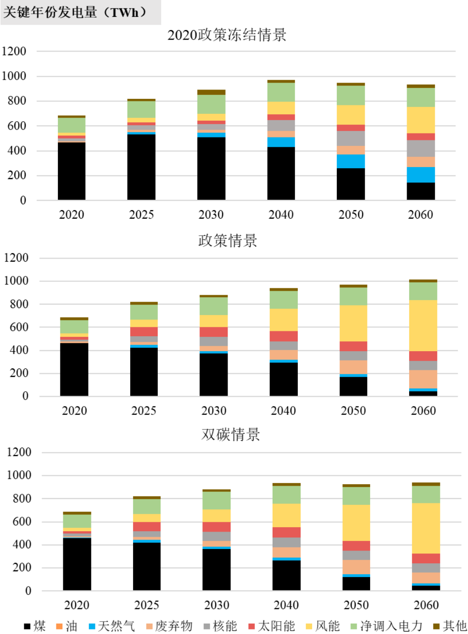
图 9 山东省关键年份发电结构
