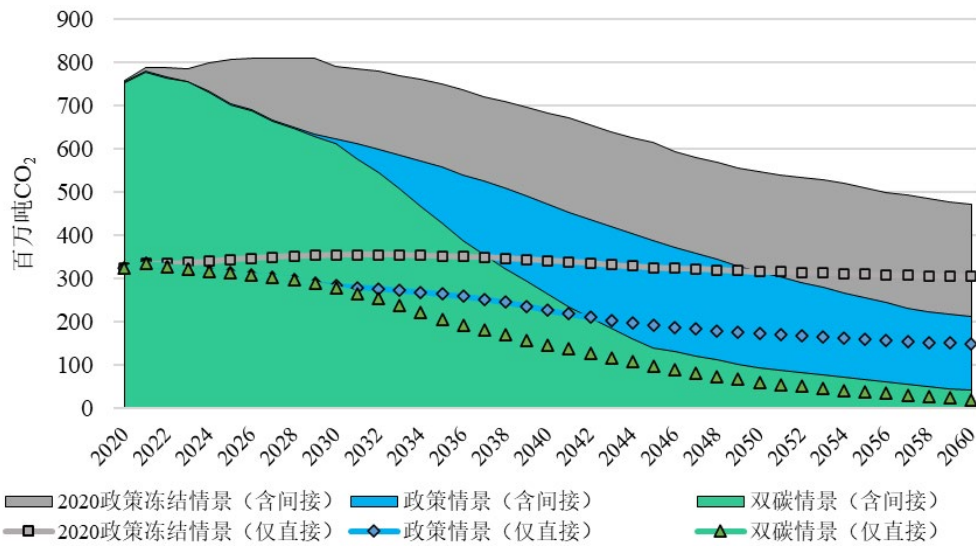
图 11 山东省工业部门碳排放趋势
