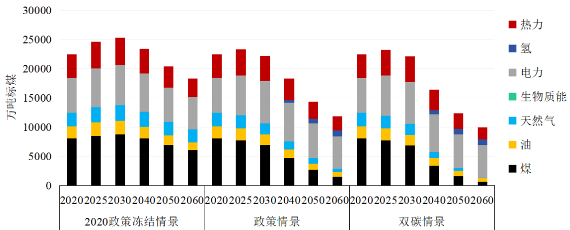
图 12 山东省关键年份工业用能结构
